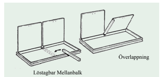
Fig 8. Dubbelluckor , plana med löstagbar mellanbalk respektive överlappning
