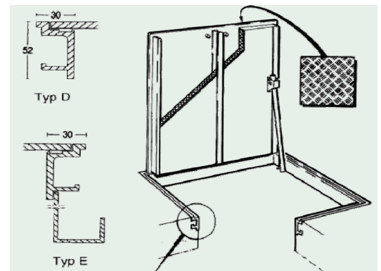
Fig 7. Enkel, plan lucka samt exempel på ramprofiler
